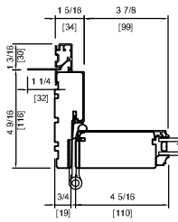
METAL CLAD DOUBLE CAMBERTOP
