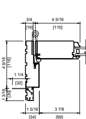
METAL CLAD DOUBLE CAMBERTOP
