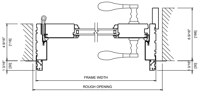
METAL CLAD 4 9/16" & 6 9/16" (116mm & 166mm)
