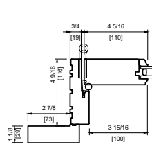
METAL CLAD DOUBLE CAMBERTOP
